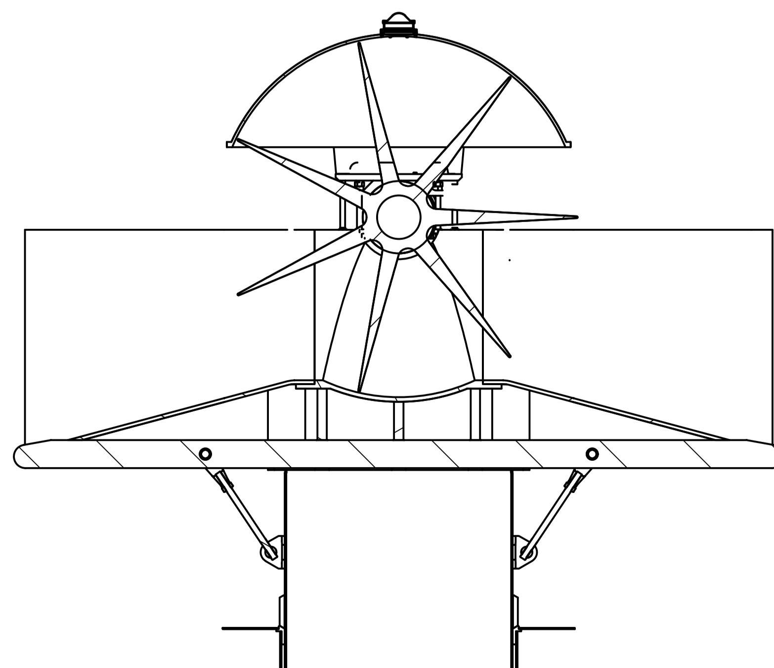
Sez A-A
